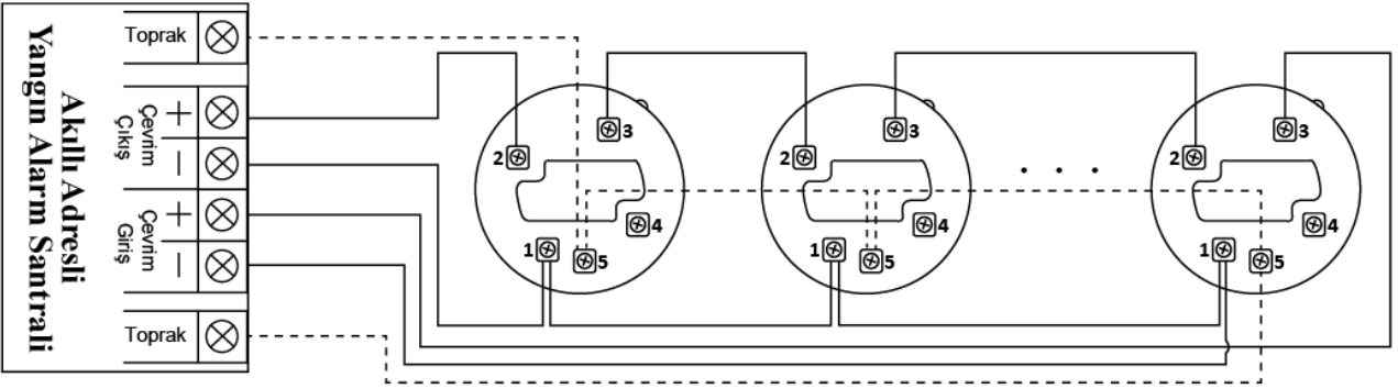
ML serisi akıllı adresli izolatörlü dedektörlerin buzzerli soket (ML-0141) bağlantı şeması
