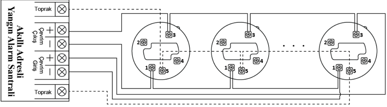
ML serisi akıllı adresli dedektörlerin buzzerli soket (ML-0141) bağlantı şeması
