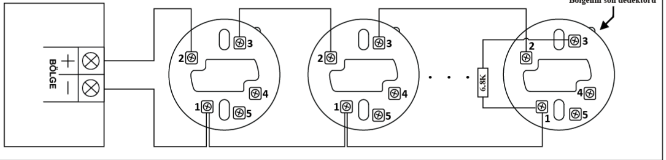
ML Serisi Konvansiyonel Dedektörlerin Buzzerli Soket (ML-0141) Bağlantı Şeması
